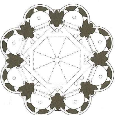
Pianta delle cucine romaniche
